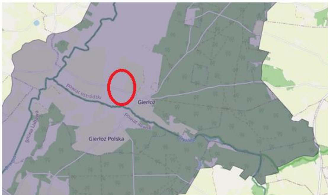
Rys. 5.7. Fragment mapy korytarzy ekologicznych Polski. Okręgiem koloru czerwonego oznaczono orientacyjne położenie obszaru opracowania. Źródło: https://mapa.korytarze.pl/
